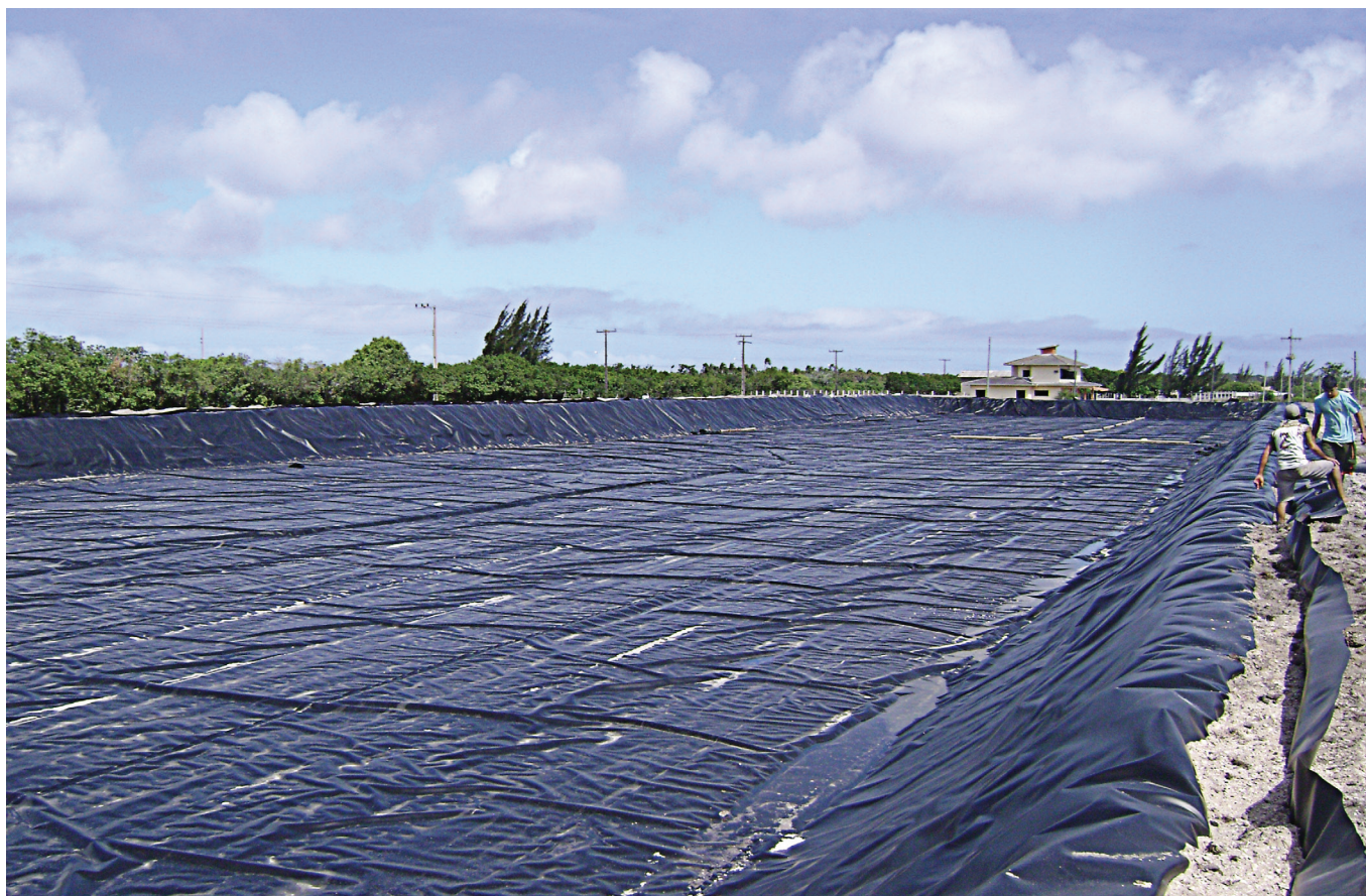
Figura 1. Revestimento do fundo do viveiro (0,6ha) com geomembrana PAD
