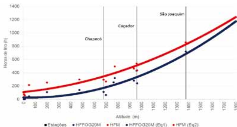
Figura 3. Horas de frio médias acumuladas de abril a setembro (HFM) em função da altitude e valor mínimo de horas de frio em que poderia ocorrer o estímulo ao florescimento em função de geadas e fenologia do mirtilo (HFFOG20M)
