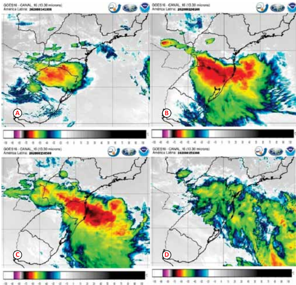
Figura 12. Imagens realçadas do satélite GOES-16 dos dias 14 e 15 de agosto de 2020, horário local: A) dia 14 às 15:00h; B) dia 14 às 22:00h ); C) dia 15 às 02:00h e D) dia 15 às 10:00h
