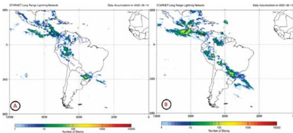
Figura 13. Descarga elétrica acumulada: A) dia 14/08/2020 e B) 15/08/2020
