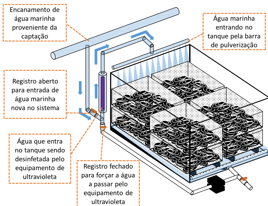
Figura 27. Enchimento do tanque com água marinha
