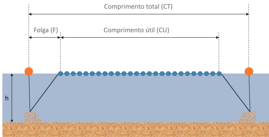
Figura 5. Esquema de fundeio de longlines
