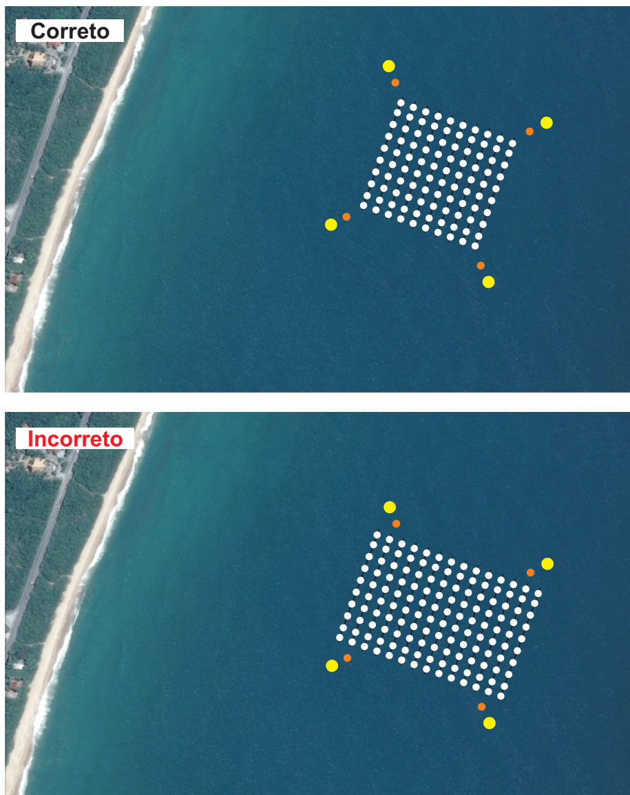
Figura 6. Recomendação de fundeio de longlines
