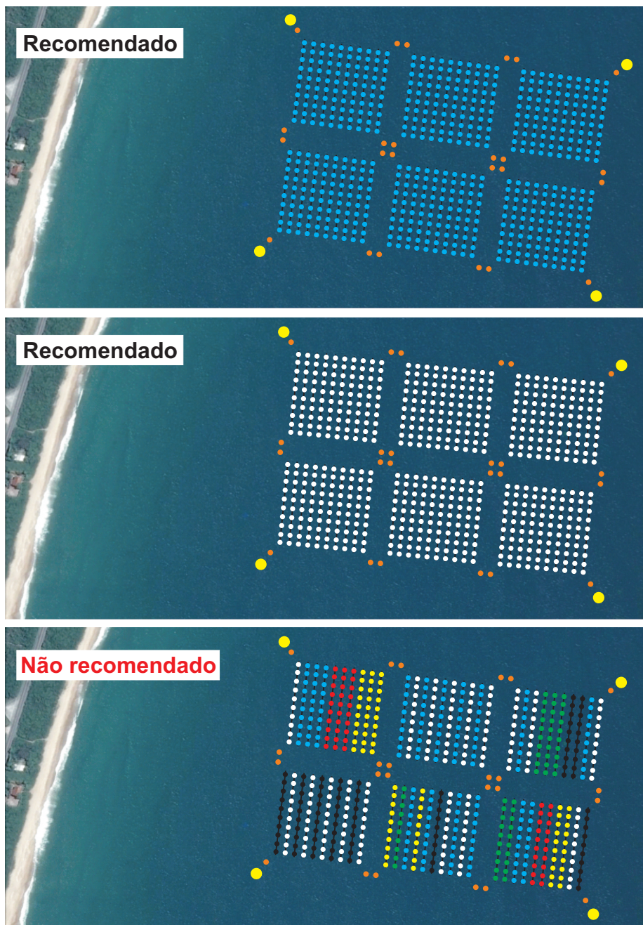
Figura 7. Padronização de flutuadores nos parques aquícolas
