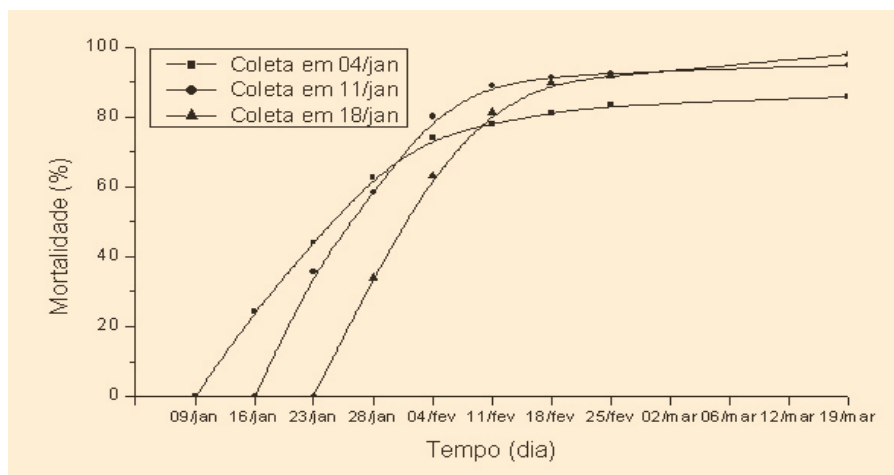
Figura 2. Progressão da mortalidade de O. oryzae infectados artificialmente por B. bassiana obtida nos ensaios executados na safra 2011/12
